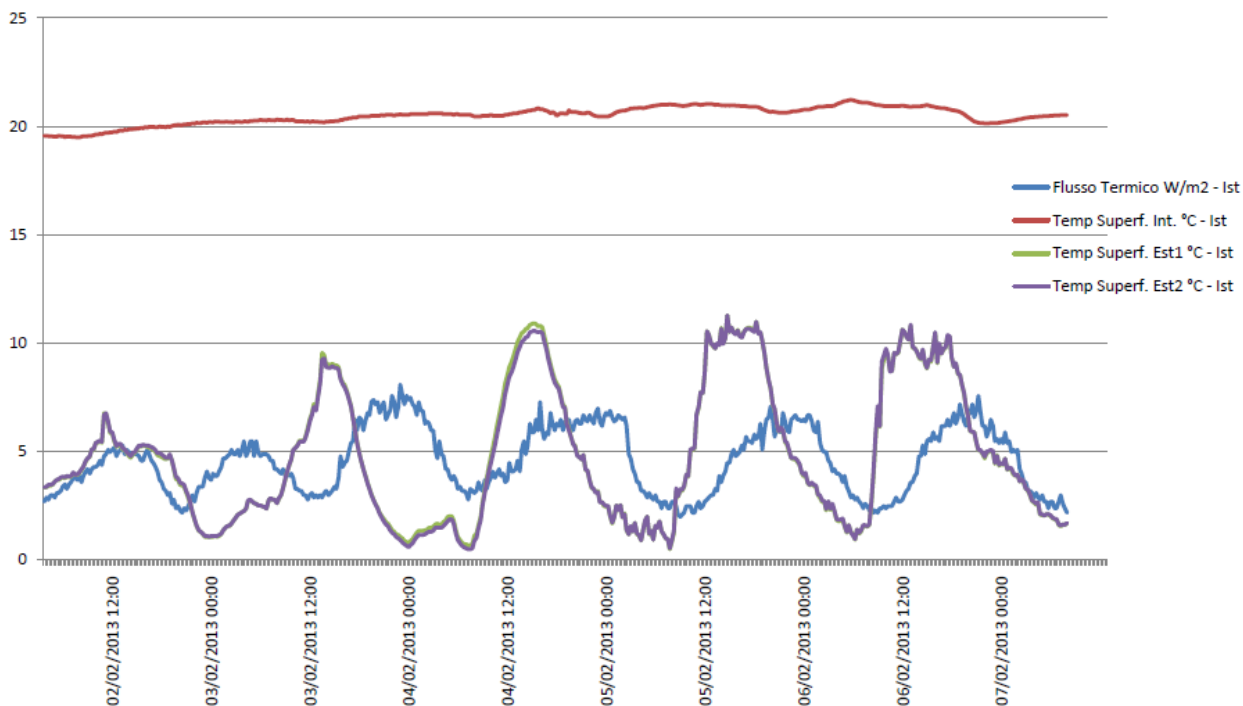
Immagine 4: Valori di flusso termico (blu), temperatura interna (amaranto) e temperatura esterna (verde e viola) misurati.
