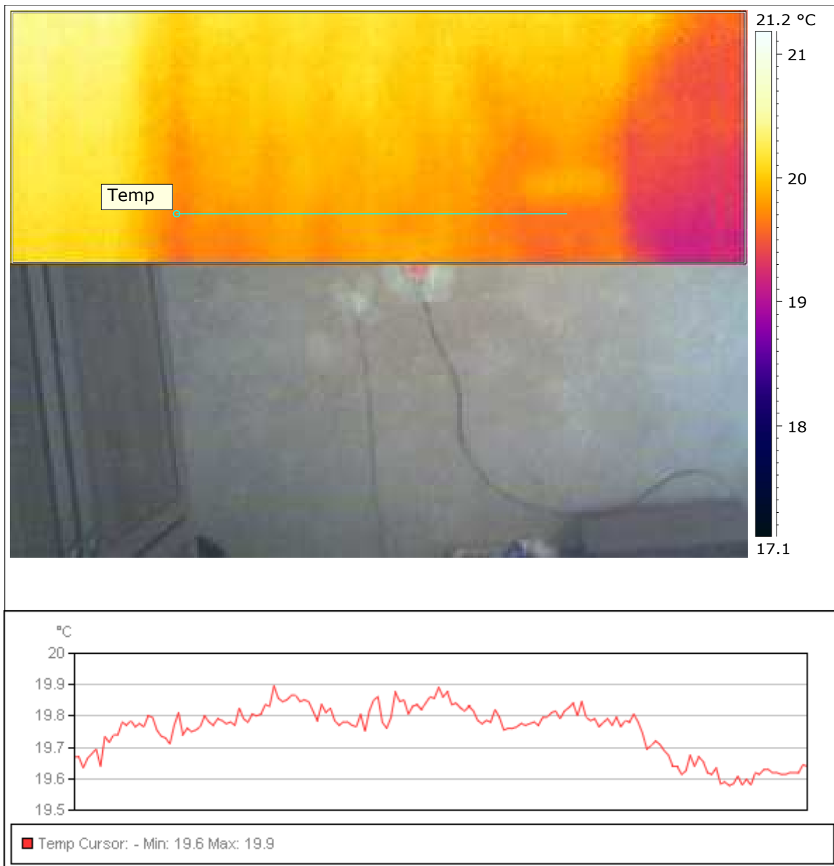
Immagine 2: Parete interna della stanza da letto matrimoniale oggetto di misura. L'immagine è ottenuta attraverso la sovrapposizione pixel to pixel della stessa ripresa nel campo ottico ed infrarosso. Si apprezza l'ottima uniformità termica superficiale come evidenziato dal grafico relativo alle temperature sottostanti la linea "Temp".
