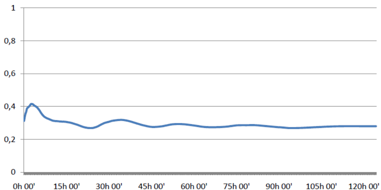
Immagine 5: Andamento nel tempo della conduttanza media. Si vede come la conduttanza tenda asintoticamente ad un prefissato valore.
